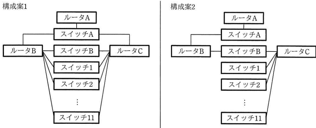
図 2 ルータとスイッチの接続形態
